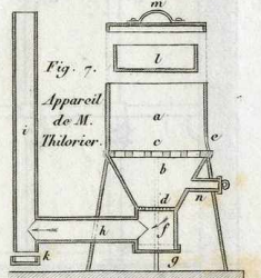
Poêle de M. Thilorier
