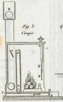
Poêle perfectionné
