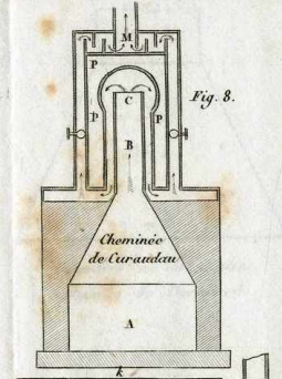
Poêle de M. Thilorier
