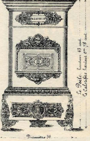
N° 6. POÈLE ou CALORIFÈRE de 1,10 mètre de hauteur de 0,75 mètre de largeur de 0,75 mètre de profondeur avec système à réservoir et bûches de chaleur de 300 à 380 Le système séparément de 50 cent de largeur de 66 cent de 120
