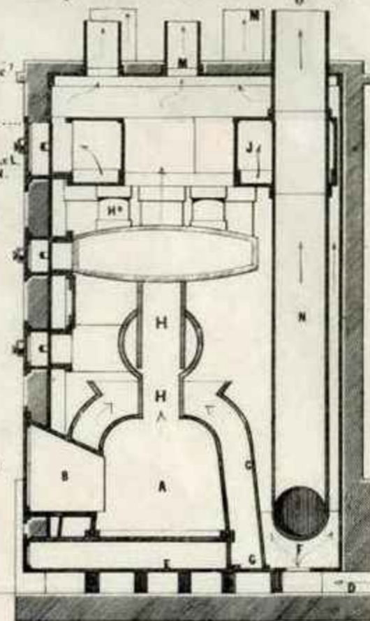
N o 4. CALORIFÈRE PORTATIF Sans galerie 125 f
