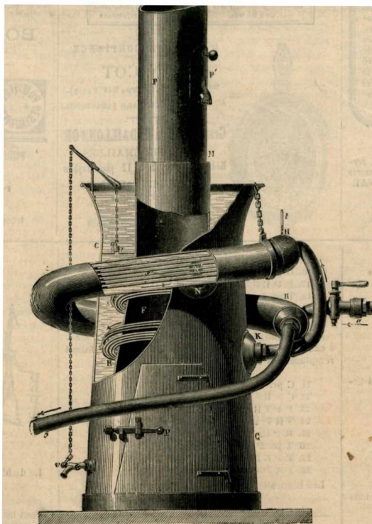
C. JULIEN. APPAREIL DE M. TERREL DES CHÊNES POUR LE CHAUFFAGE DES VINS. Gravure extraite des Études sur le vin , par M. Pasteur. (Librairie F. Savy.)
