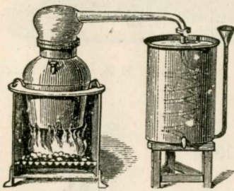
Alambic-brûleur pour la distillation simple des matières pâteuses, marcs et lies.
