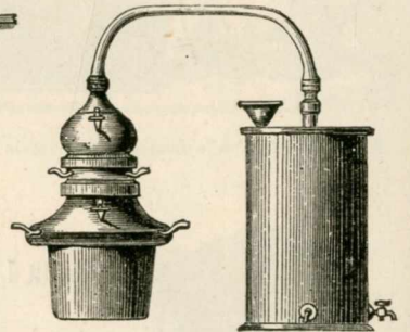
Alambic vendu d'après la contenance du bain-marie.
