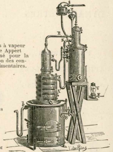
Appareil ÉGROT, petit modèle, vendu avec fourneau et trépied.
