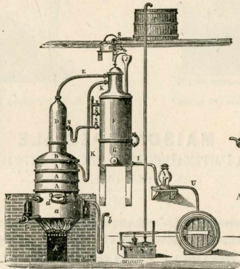
Alambic-brûleur pour la distillation simple des matières pâteuses, marcs et lies.
