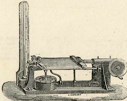
Machine d'essai pour papiers et tissus.
