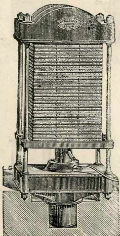
Presse à froid pour stéariniers. Charge 400 pains.
