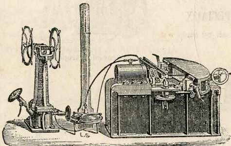
Machine d'essai à la flexion. Force totale : 50 tonnes.
