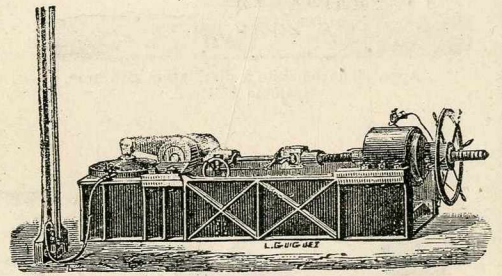
Machine d'essai à la traction. Types de 25, 50 et 100 tonnes.
