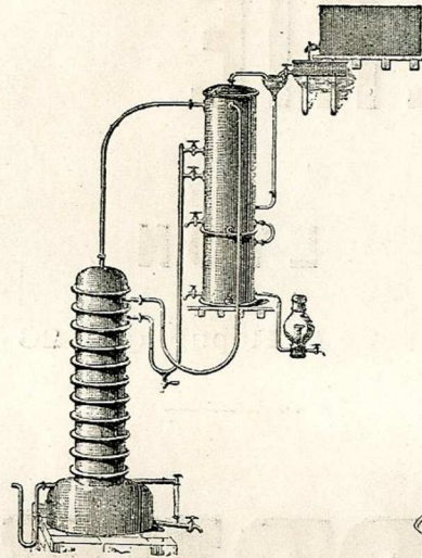
Appareil à distiller tous les jus fermentés.
