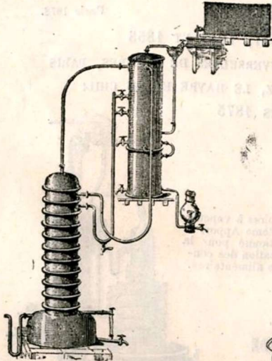
Appareil à distiller tous les jus fermentés.
