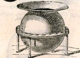
Chaudière à double fond pour teinturier.
