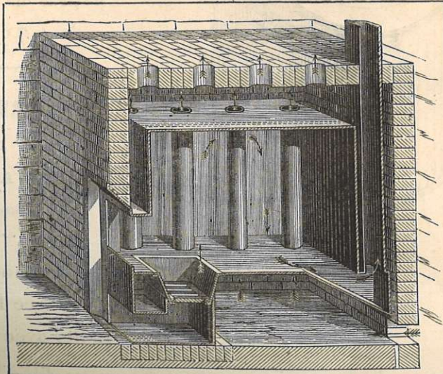
CALORIFÈRE DE CAVE rendant toute la chaleur produite par le combustible.
