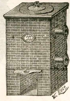
CHAUDIÈRES MAÇONNÉES POUR THERMOSIPHONS Point de surveillance de nuit
