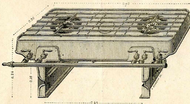
Vue du même Réchaud baissé, pour le service des feux du dessus et de la grillade.
