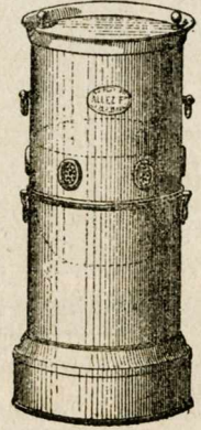
Brazéros en tôle avec sans roulettes garniture cuivre à l'usage de la braise, sans tuyau.
