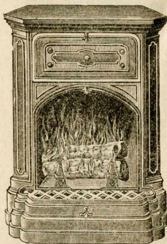
Cheminée à socle , avec four, foyer terre réfractaire au bois, tuyau dessus ou derrière. Hauteur. . . . . 0.73 0.79 0.85 Largeur. . . . . 0.61 0.65 0.71
