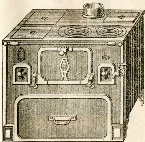
Fourneau américain. 2 réchauds à charbon de bois, réservoir à eau chaude avec panache et couvercle cuivre, à arcade avec ou sans charbonnier.
