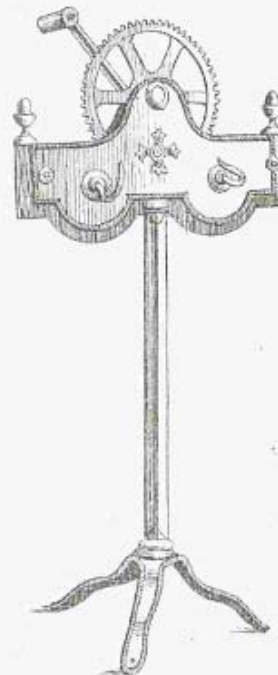
Machine à fabriquer les liens
