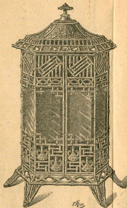
N° 3054 (Hexagone allongé) Bambou Hauteur totale ..... 0 m 96 Long r de la base 0 m 56 - Larg r de la base 0 m 38 Prix Verni ..... 50 fr. Email vert 68 fr.
