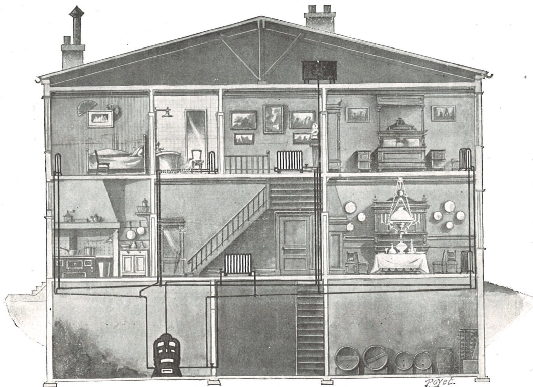
Vue en coupe d'une habitation montrant la position de la chaudière et des radiateurs et la distribution des tuyaux.
