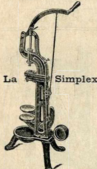
Machines à boucher, à compression latérale. La Simplex.. 33.50 La Française.. 35. » La Meilleure.. 35. »
