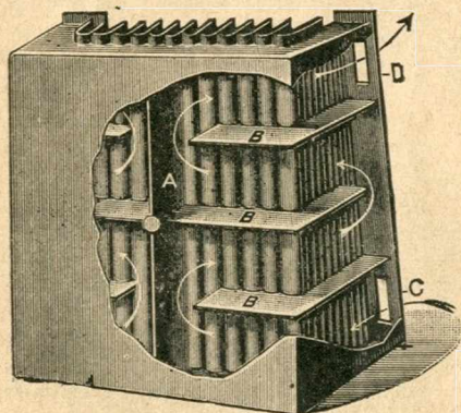
VUE DE DOS Montrant le parcours de l'air chaud.
