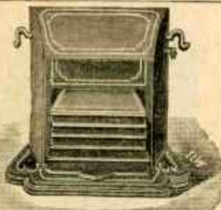
Foyer économique, terre réfractaire avec un souffleur, dessus oblique au charbon.
