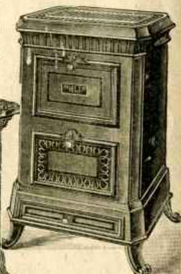
Cheminée de salle à manger Godin, à four, couvercle à charnières, foyer terre réfractaire au bois et au charbon, tuyau derrière.
