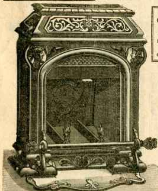
Cheminée style moderne, modèle riche, foyer à bois, intérieur briques réfractaires qui reçoivent directement la chaleur et l'emmagasinent. L'air entrant par des bouches ménagées dans le bas de la cheminée, circule autour de ces briques et se répand dans la pièce par des bouches placées à la partie supérieure. Tuyau derrière et ovale. Haut. 0 m 90. — Larg. 0 m 82. — Profondeur du foyer 0 m 33. Largeur du foyer 0 m 44. Fonte vernie, garniture nikelée. . . . . 142. » Email noir avec garniture nikelée . . . . . 154. »
