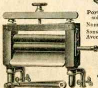
Essoreuse, monture bois, rouleaux caoutchouc, à vis de pression, se plaçant sur un baquet.
