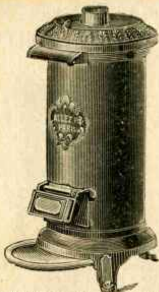
Calorifère Godin, tôle et fonte, sans grille, tuyau dessus ou derrière, intérieur briques réfractaires au coke. Haut. 0 m 52 0 m 57 0 m 65 0 m 75 Prix. 12.35 15.20 18.15 21.85 Haut. 0 m 84 0 m 91 0 m 97 1 m 20 Prix. 25.65 34.20 43.70 49.40 (Se fait avec couvercle pour brûler le bois. Même prix, tuyau derrière).
