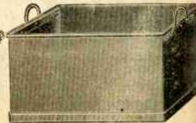
Boîtes à ordures, série forte, peinte. 53x32 65x42 75x45 Contenance, 40 lit. 80 lit. 120 litres. Prix . . . . . 5.50 8. » 10.50 Galvanisées, 6.50 9.50 12. »
