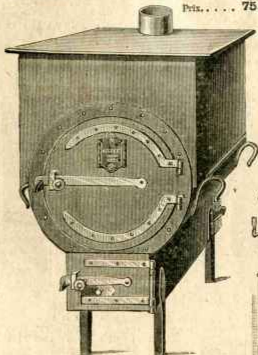
Four forain, pour pâtisserie.
