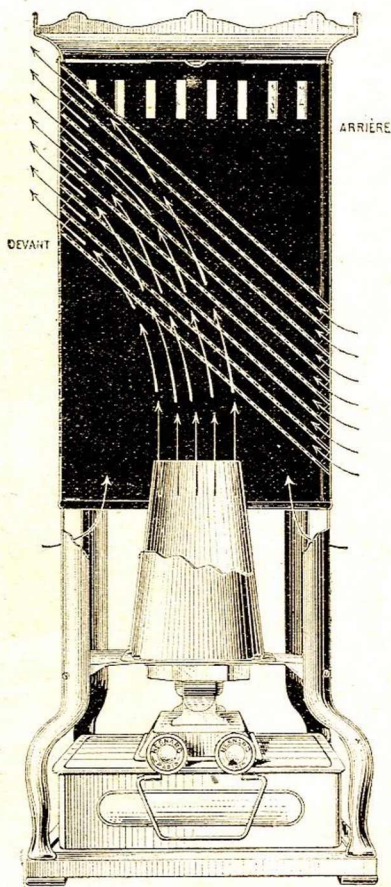
Coupe du dispositif de chauffage du Calorifère “ BRULE-BLEU ” (1).
