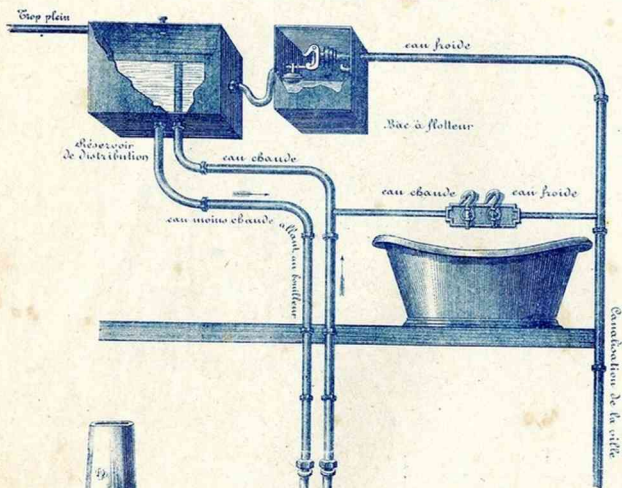
Schéma de l'installation d'un bouilleur desservant une salle de bains
