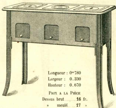
N° 25. — A TROIS TROUS
