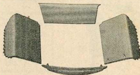
FOTER DÉCOMPOSÉ EN 4 PIÈCES POUR CHAUFFAGE A LA HOUILLE
