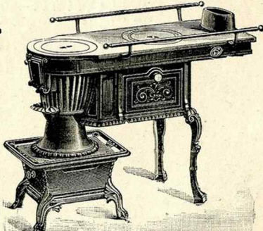
N os 31 ET 32, avec porte au foyer sur demande
