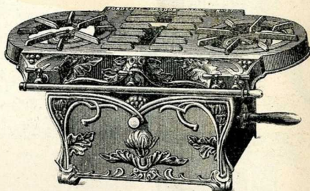
Dimensions du four : 0 m 32×0 m 32
