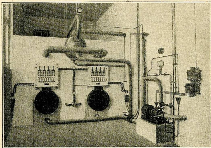
Chauffage centra lélectrique d'une usine
