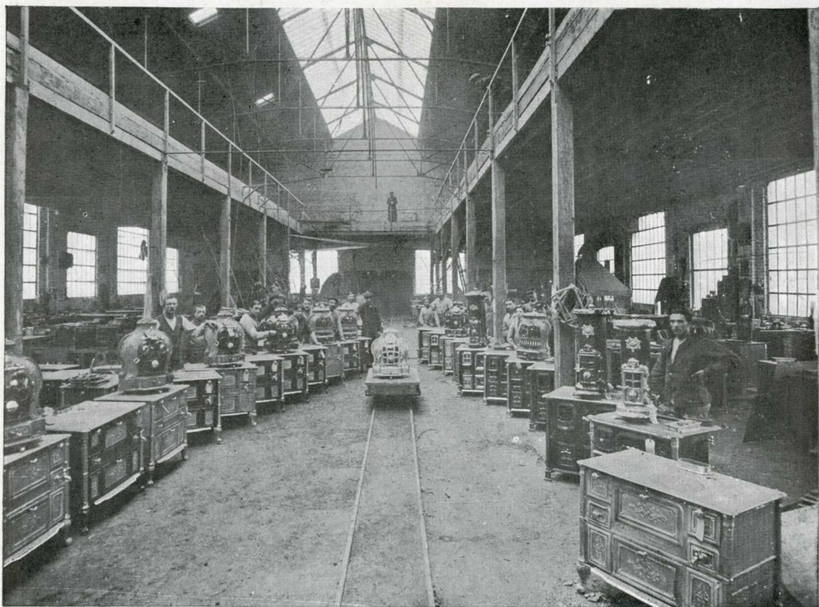
En haut : les ruines d'une des usines. En bas : le nouvel atelier de montage des cuisinières en tôle émaillée.
