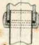
Fig. 2 Coupe d'un joint à bague
