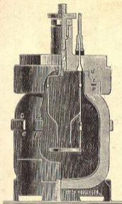
Bombe Calorimétrique
