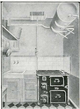
Appartements à Paris, chauffés par Fourneau "IDEAL CULINA et 4 Radiateurs. Installation faite en 1926. Prix : Frs 5 200 y compris la distribution d'eau chaude.
