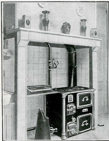
Maison à Duclair (Seine-Inf.), chauffée par Fourneau "IDEAL CULINA" et 3 Radiateurs.
