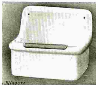
Fig. 1999 — Vidoir grès de face, hauteur 38, largeur 45, saillies 31, profondeur 16. Prix, ... Classe A, Fr. 320. » B, Fr. 240. » D'angle, même prix.
