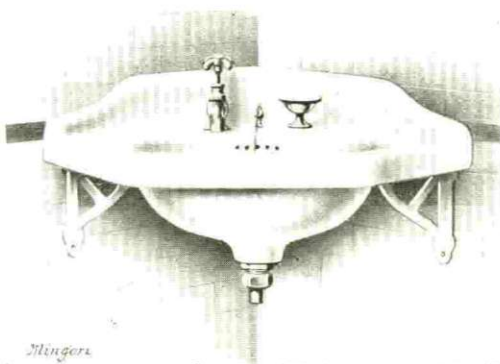
Fig. 1910. — LAVABO D'ANGLE. Avec bonde à bouchon, 1 robinet, 1 baignier, consoles en fonte peinte 62×46 Fr.... A 270 " B 245 " 68×50 Fr.... A 310 " B 245 " Plus-value pour vidage à bascule en 68×50 Fr..... 80 "
