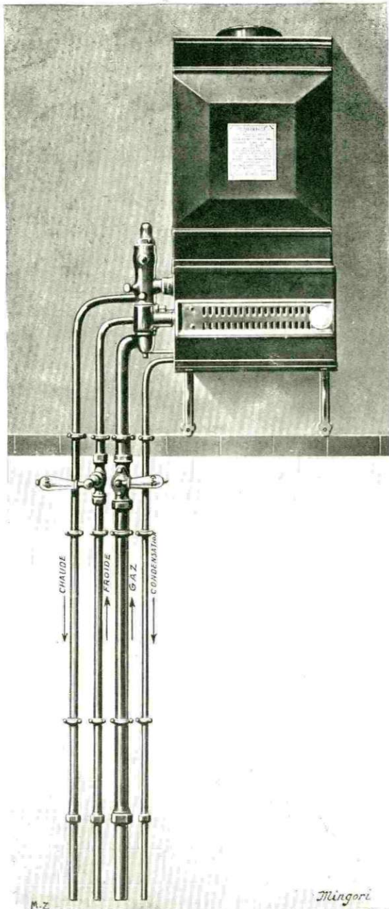
CHAUFFE-BAINS au gaz à pression monté avec valve automatique ci-contre, fig. 6000 à 6004 bis. (Voir tarif 7, page 7, paragraphes 1 et 2.)
