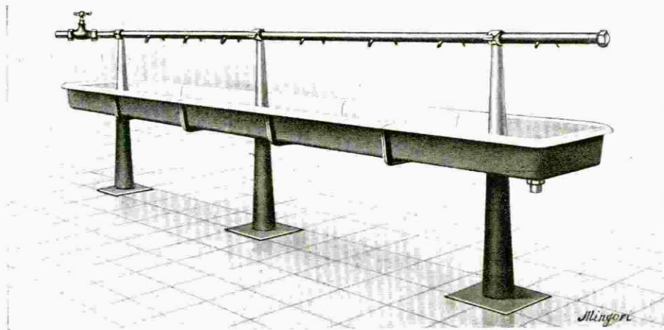
Fig. 9010. Hauteur du sol au bord supérieur 91 1 / m , largeur du Lavabo 72 1 / m , creux 20 1 / m , diamètre prévu pour tuyau de distribution 60 1 / m . NOTA. — Le tuyau de distribution d'eau n'est pas livré, sauf sur demande. (Voir tarif 7, page 27, paragraphe 41).
