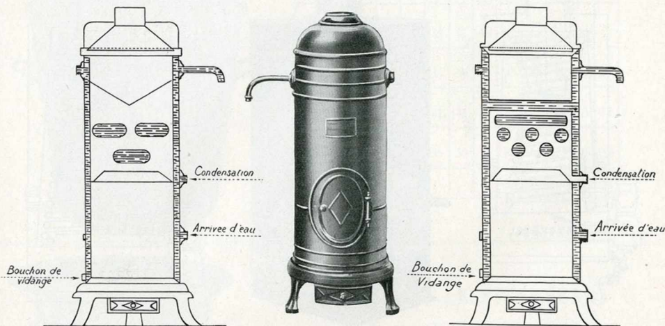
Coupe du chauffe-bain 605, 12 litres
