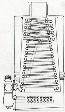
Coupe des Chauffe-bains 608, 608 bis, 614, 614 bis
