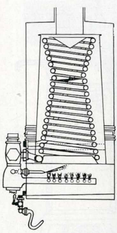
Coupe des Chauffe-bains 607, 607 bis, 611, 611 bis
