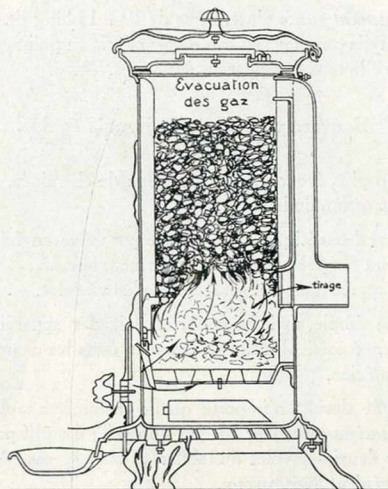
Coupe d'un calorifère à feu visible et continu.
