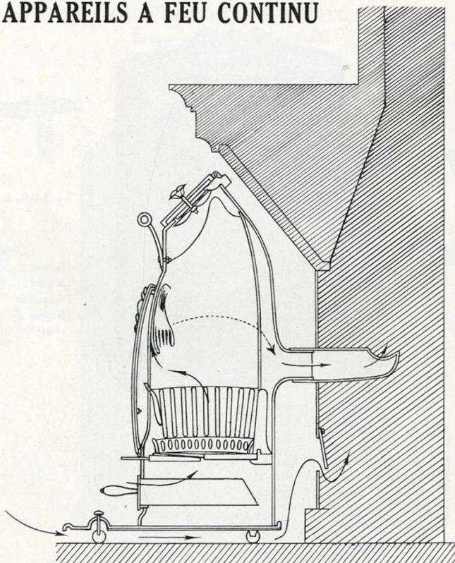
Coupe d'un appareil à feu continu.
