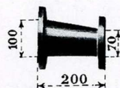
Raccord de réduction.
