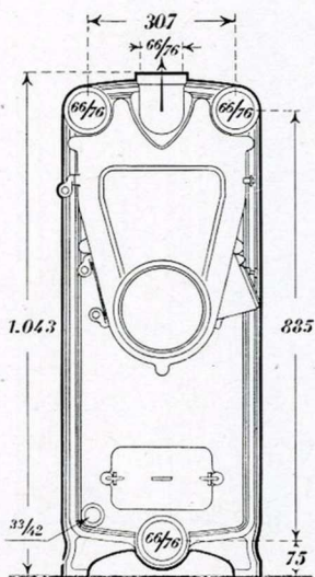
Chaudière avec buse de fumée à l'arrière.
