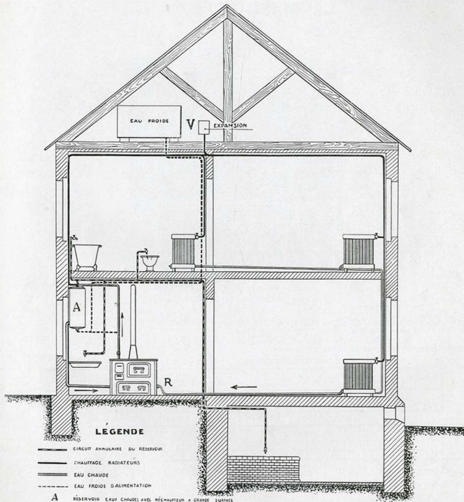
SCHEMA D'UNE INSTALLATION ORDINAIRE DE CHAUFFAGE CENTRAL
