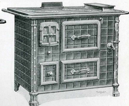
Vue d'une cuisinière N° 5511 avec barre contourante, porte de foyer à mica, chaudière avec panache dessus avec 2 flottes mobiles.
