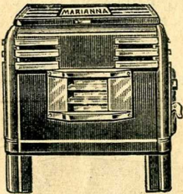
78-P-362. POËLE à bois Deville Marianna , tout en fonte émaillée céramique gris-bleu, bleu ou marron, garnitures nickelées, sol réfractaire, réglage par ventouse à vis.
