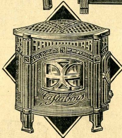
78-P-363. POËLE à bois Taftabois , tout en fonte émaillée céramique toutes teintes. Couvercle à charnière, sol réfractaire, réglage par ventouse à vis et clef de manœuvre. Sans précédent.....
