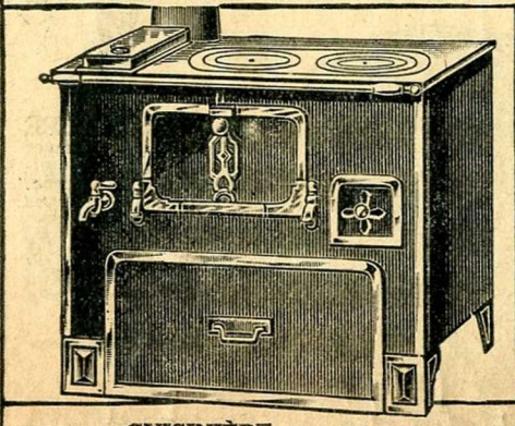
78-P-317. CUISINIÈRE tôle et fonte, à charbonnier et retour de flamme. Sans chaudière. Largeur 0=70, tuyau de fumée à droite ou à gauche. 295. La même, avec chaudière fonte émaillée. 345.
