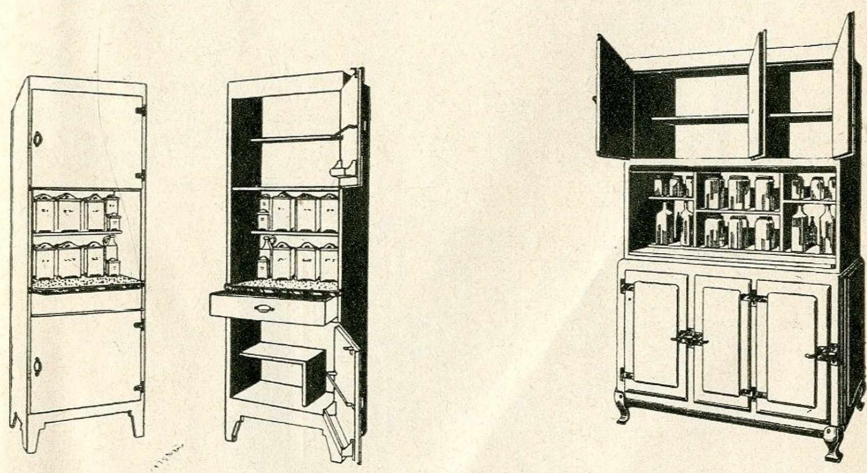
Buffet américain, petit modèle Long. 0,60, larg. 0,45, haut. 1,815
