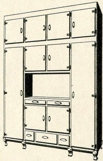
Buffet américain avec table à éclipse Avec annexe A ou B, long. 1,37, larg. 0,47, hauteur 1,95. Avec annexes A, B, C, long. 1,84, larg. 0,47, hauteur 2,50.
