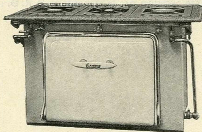
Réchaud-Four N° B 70 (5 robinets)
