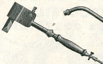
FER A SOUDER "RAPIDE" AU GAZ BUTANE
