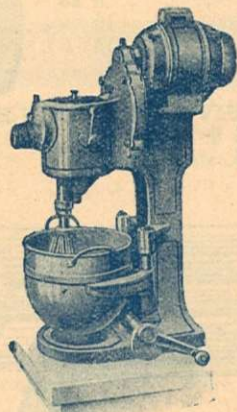
Modèle E , avec moteur \frac{1}{6} cv. courant triphasé
