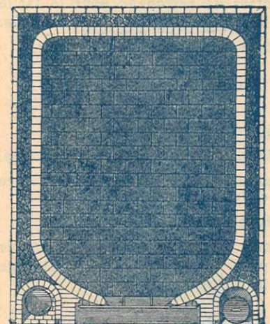
Plan de la Sole d'un Four
