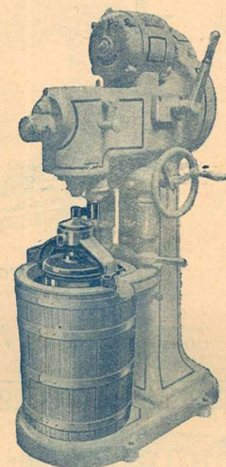
BATTEUR-MELANGEUR équipé avec une sorbetière.
