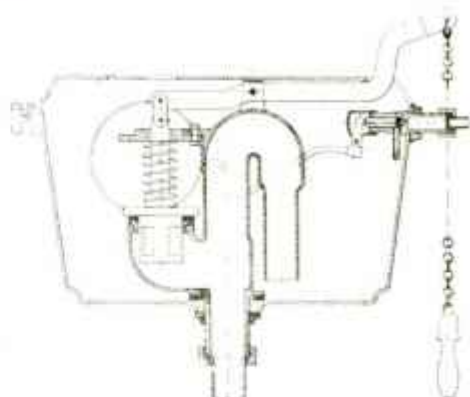
Coupe du réservoir à clapet n° 1330.
