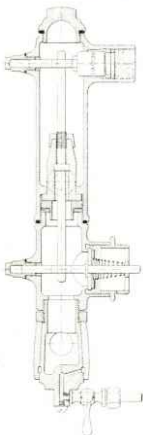
Coupe du distributeur d'eau chaude "Le Coq"
