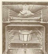
Rampe pour griller avec plafond rayonnant à picots
