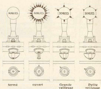
Flamme aux différentes positions.
