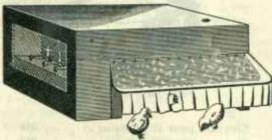
ELEVEUSE OUVERTE « CC » au début de l'élevage.
