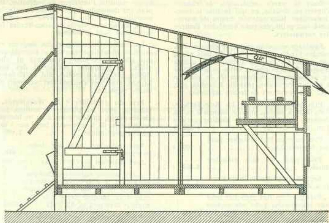
Dessin-coupe montrant le système d'aération du poulailleur américain Amblard dénommé « Maison pour Poules ».
