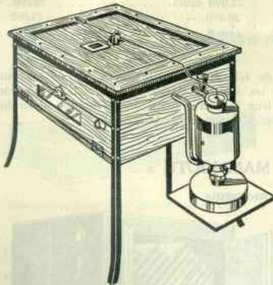
Couveuse-séchouse à thermo-siphon 120 œufs.
