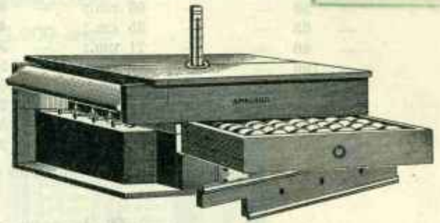
COUVEUSE « CS » s'ouvrant pour le retournement des
