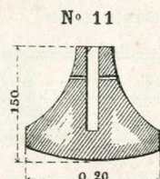
Poids : 12 kil.
