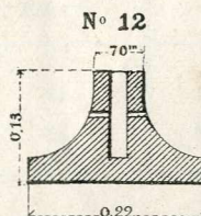
Poids : 11 kil.
