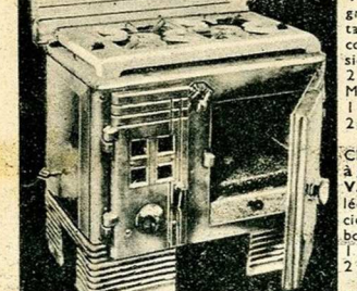
CF-25.631. RÉCHAUD à gaz de pétrole "B. H. V.", bâti fonte émaillée granitée, bec silencieux, réglables à débouchage automatique. 1 feu..... 140.» 2 feux..... 245.» Marque "Cobra"..... 1 feu..... 180.» 2 feux..... 270.»
