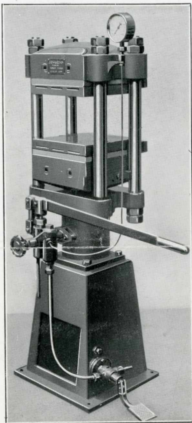
PRESSE N° 1 bis chauffante à l'électricité
