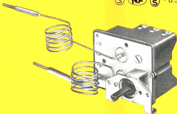
Bipolaire avec sécurité tripolaire 30 A.
