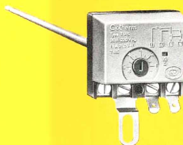
Unipolaire avec sécurité 20 A.
