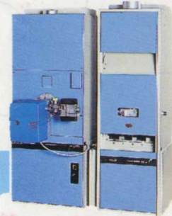
GENERATEURS D'AIR CHAUD SERIE RESIDENTIELLE Fuel et Gaz de 10 à 60 Kw 7 modèles
