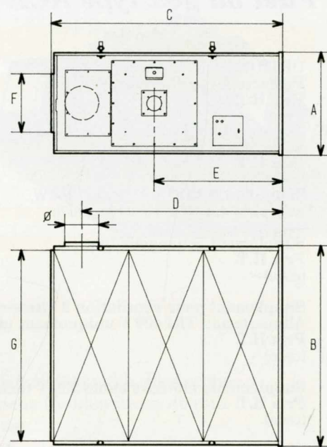
Générateur "couché gauche"
